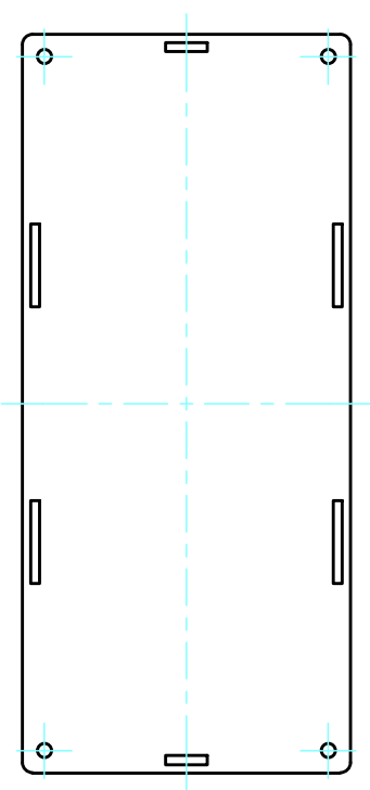
下カバー表面 / Bottom cover Frontside
