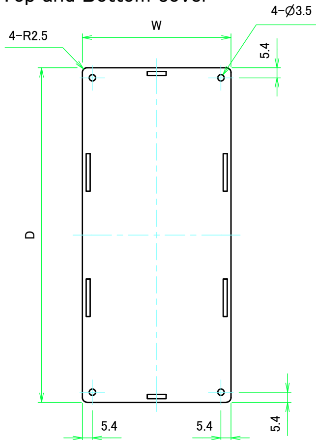
上カバー表面 / Top cover Frontside
